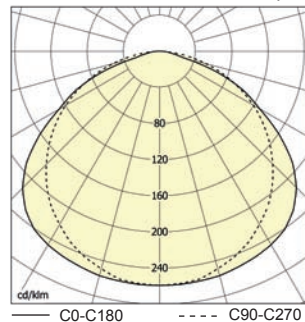
FARGO, 2x58W, IP65 - Festett acél fényterelő
